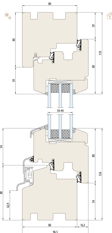
SV-Hout 80 met triple glas
