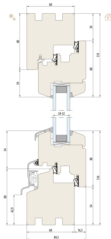
SV-Hout 68 — verticale doorsnede
